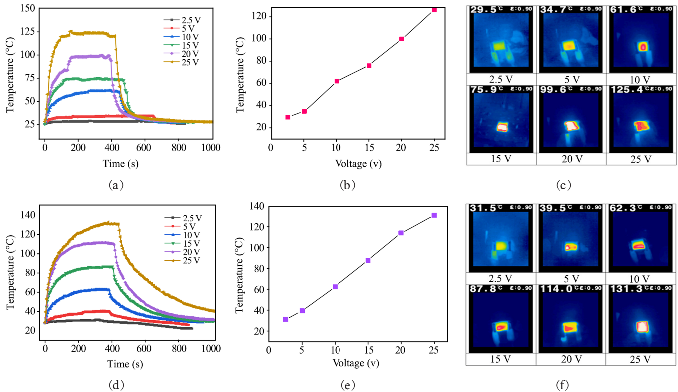
شکل ۷- نمودار تغییرات دما برحسب زمان، نمودار دمای اشباع برحسب ولتاژ و تصاویر دوربین زیرقرمز در ولتاژهای مختلف برای پارچه‌های حلقوی (a)-(c) پنبه/پلی‌آنیلین و (d)-(f) پنبه/پلی‌آنیلین/مکسین.
