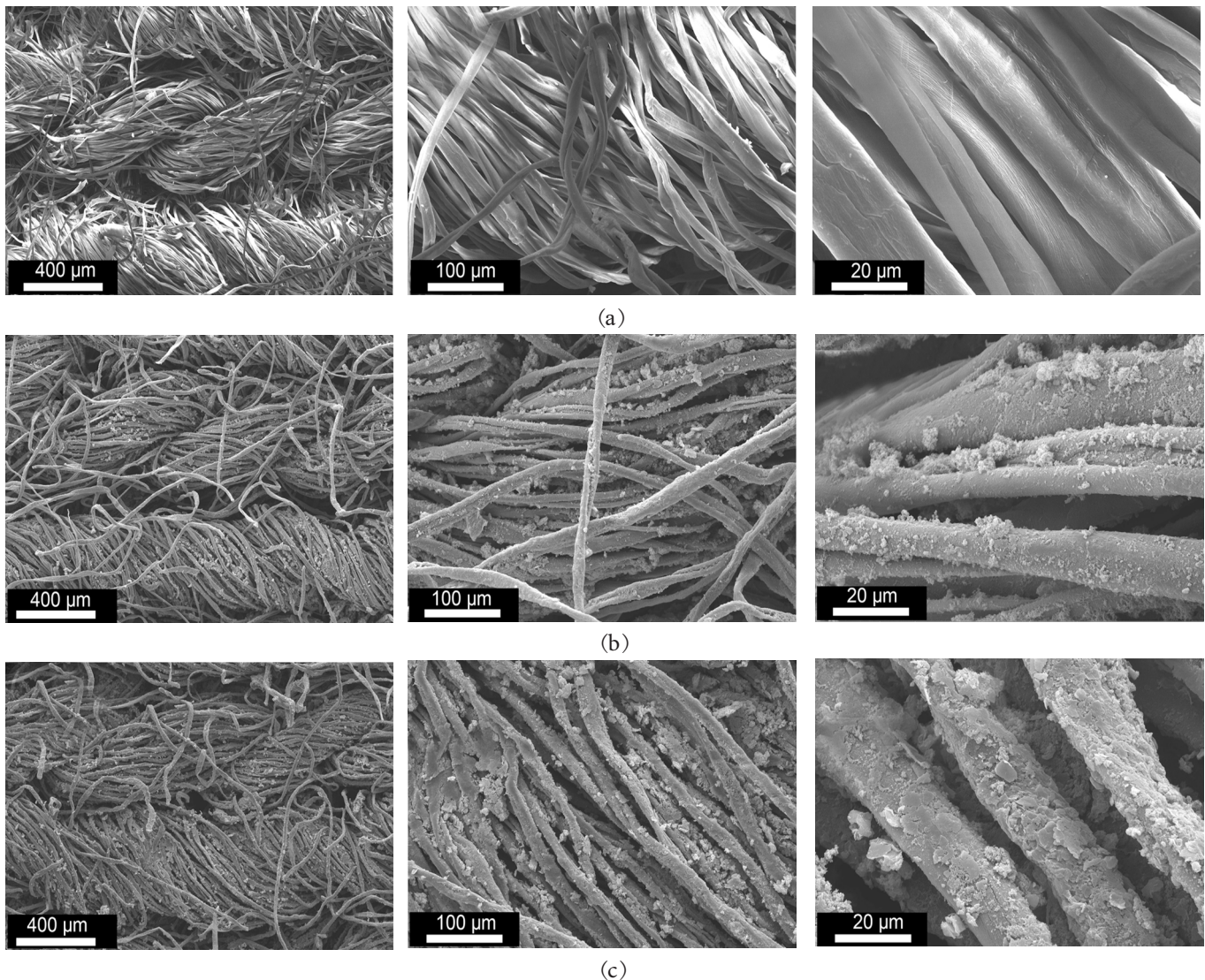
شکل ۵- تصاویر FE-SEM با بزرگ‌نمایی‌های مختلف پارچه‌های (a) پنبه، (b) پنبه-پلی‌انیلین و (c) پنبه-پلی‌انیلین/مکسین. Fig. 5. FE-SEM images at different magnifications of (a) cotton, (b) cotton/polyaniline, and (c) cotton/polyaniline/MXene fabrics.
