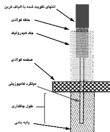
شکل ۳ نمایی از روش بکار گرفته شده برای ارزیابی چسبندگی میلگرد به بتن.
